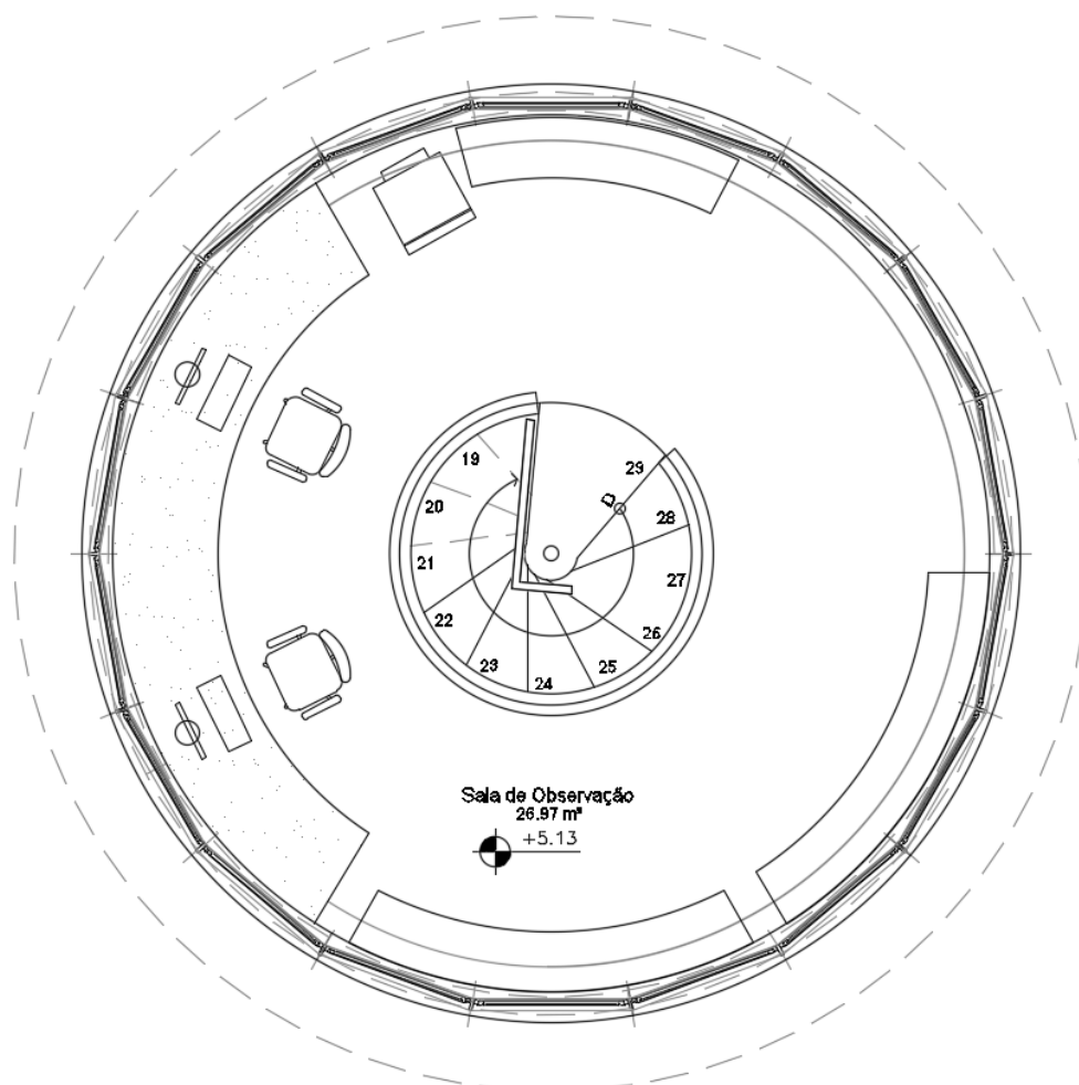
Figura: Pavimento Superior (Sala de Observação) da Torre de Observação
