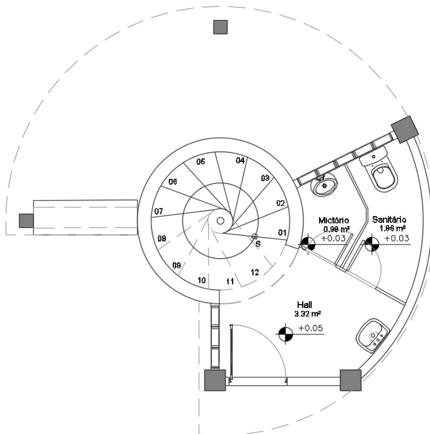
Figura: Planta Baixa do Pavimento Térreo
